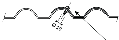
Recouvrement 1 onde et coutureage
